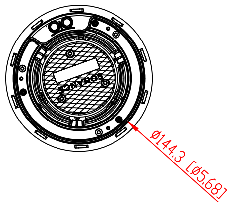
TRIMLESS GRILLE
